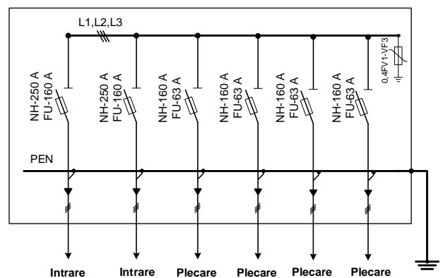
nr. 6. Schema monofilară a cutiei de cablu cu 6 aparate de comutație
